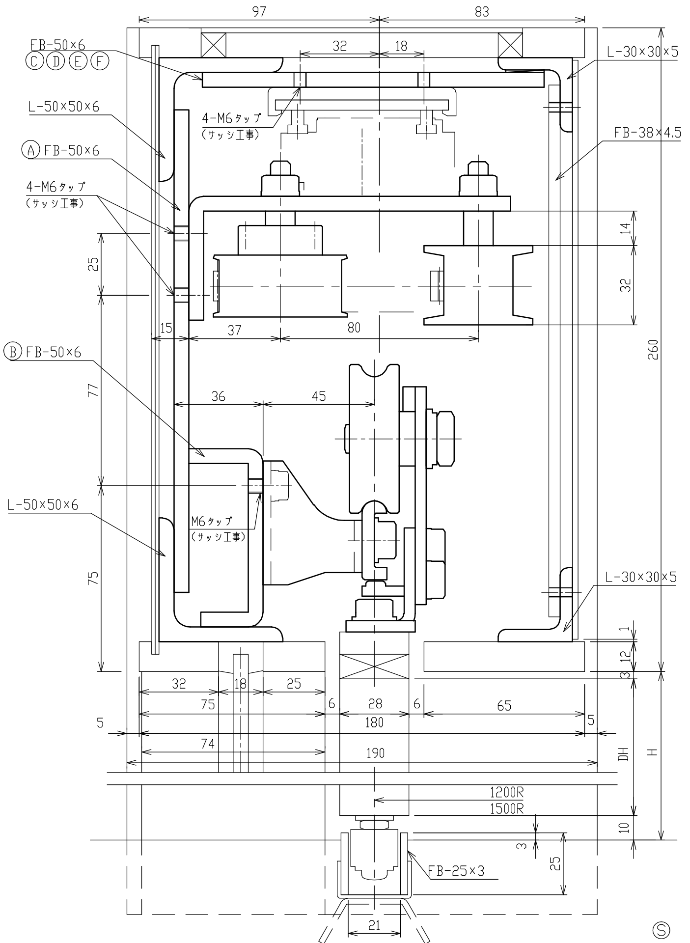
円形ドア納り 1200R・1500R SOT-R200 両引き 図番8-2 たて断面図
